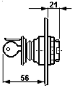
Schlagastervorsatz "NOT-AUS" mit Schlüsselentriegelung
