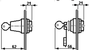
Schlüsselschalter*/ tastervorsatz
