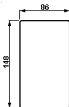
Gabarit de perçage pour GHG 412 82
