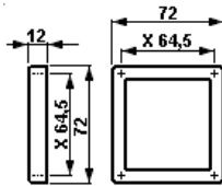
Tête d'instrument de mesure AM 72
