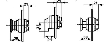
Bouton-poussoir coup de poing "ARRÊT D'URGENCE" Interrupteur + Potentiomètre Bouton-poussoir coup de poing
