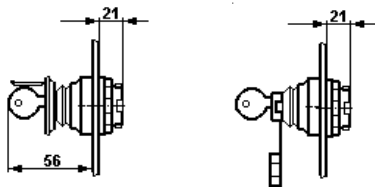
Schlagtaster "NOT-AUS" mit Schlüsselentriegelung
