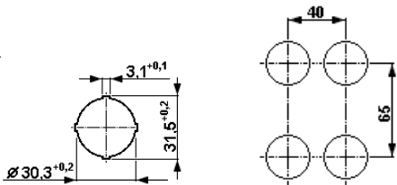
Perçage pour éléments de commande
