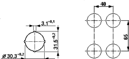
Bohrung für Bedienelemente
