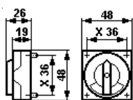
Tête de commutateur de commande Ex 23
