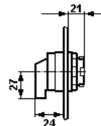
Tête de commutateur de commande et de potentiomètre *1
