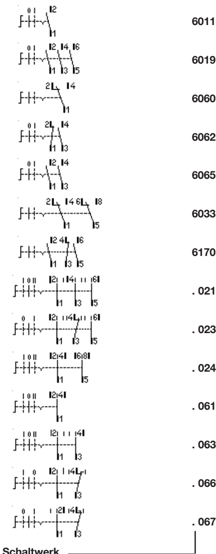
Bild 1 Anschlussbilder Steuerschalter Ex 23/Ex 29
