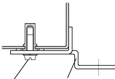
Bild 2 Wandbefestigungslasche
