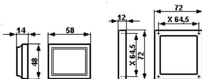
Instrument de mesure AM 45 AM 72
