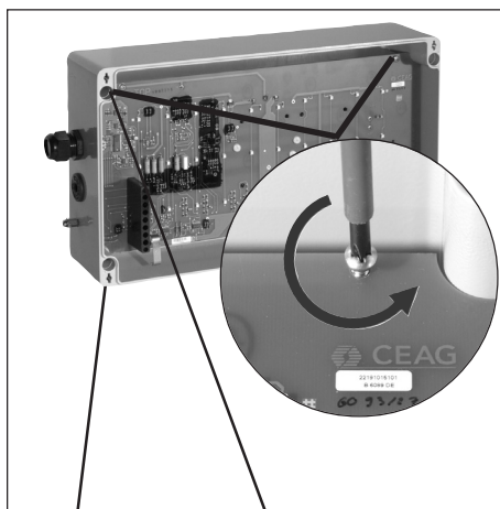
Bild 1/fig. 1/Fig.1 Befestigungsschrauben/ Fixing screws/ vis de fixation Ø 5 mm
