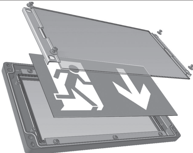
Bild 5/fig. 5/Fig. 5 Wechsel der Piktogramm-Scheibe/ Changing of legend-mask/ Replacement de pictogramme Modification du calibre de pictogramme
