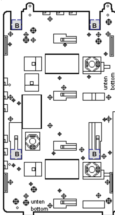
B = Steckbefestigungspunkte für Steuerschalter D22 293
