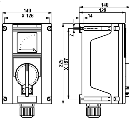
Steuerschalter D22 293, mit Messinstrument für Wandleran- schluss
