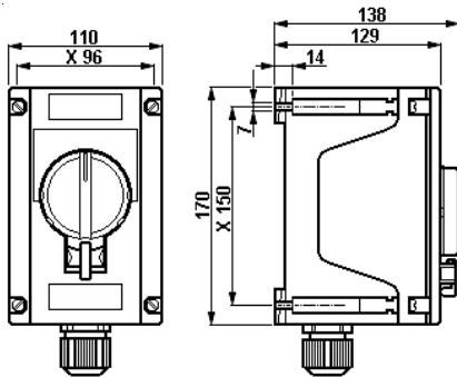
Steuerschalter D22 292
