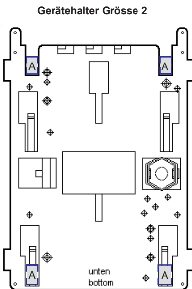
A = Steckbefestigungspunkte für Steuerschalter D22 292
