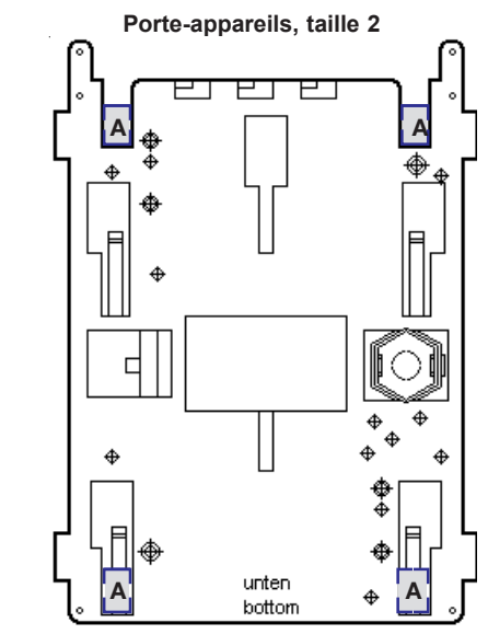
A = points de fixation pour commutateurs de commande D22 292
