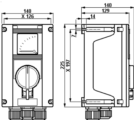
Commutateur de commande D22 293, avec instrument de mesure à lecture directe
