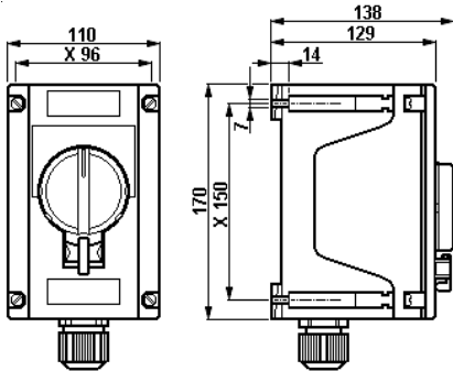
Control switch D22 292
