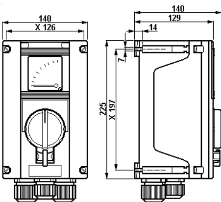
Steuerschalter D22 293, mit Messinstrument für Direktan- schluss
