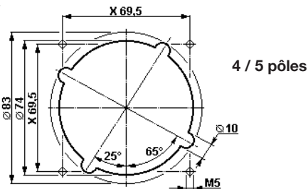
Gabarit de perçage pour prise à bride
