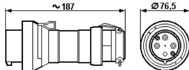
Fiche à 4 pôles
