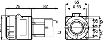
Prise à bride à 3 pôles
