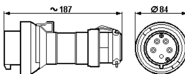
Stecker 5-polig
