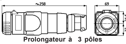
Prolongateur à 3 pôles
