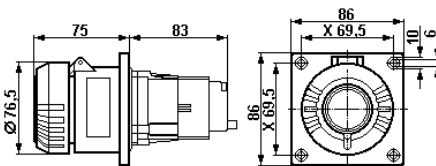
Prise à bride à 4 pôles
