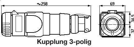
Kupplung 3-polig
