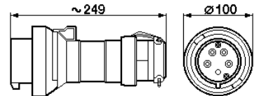
Stecker / Plug / Fiche GHG 512 75 4-pol./pôl. + PE
