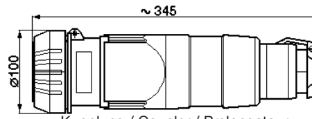
Kupplung / Coupler / Prolongateur 4-pol./pôl. + PE
