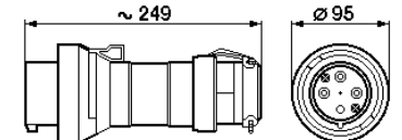
Stecker / Plug / Fiche GHG 512 74. 3-pol./pôl. + PE
