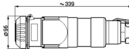
Kupplung / Coupler / Prolongateur 3-pol./pôl. + PE
