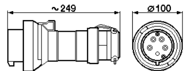
Stecker / Plug / Fiche D22 517 75 4-pol./pôl. + PE
