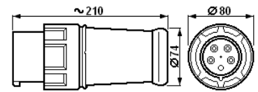
Stecker / Plug / Fiche D22 532 7. 3/4-pol./pôl.+PE
