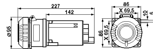
Flanschsteckdose/Flange socket/Prise à bride 3-pol./pôl. + PE
