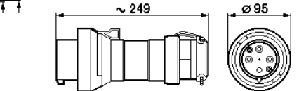
Stecker / Plug / Fiche D22 517 74. 3-pol./pôl. + PE
