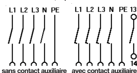
D22 518, 5 pôles 50/60 Hz
