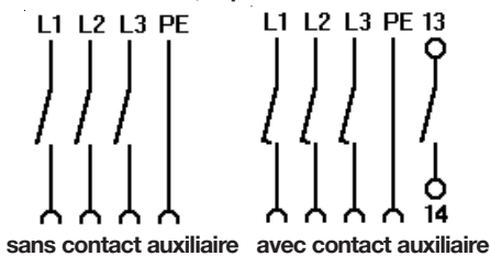
D22 518, 4 pôles 50/60 Hz
