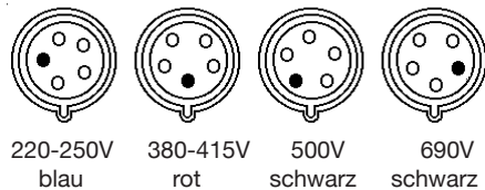
D22 518, 5-polig 50/60Hz
