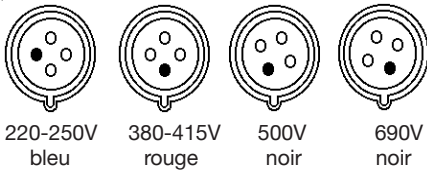
D22 518, 4 pôles 50/60Hz
