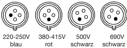
D22 518, 4-polig 50/60Hz
