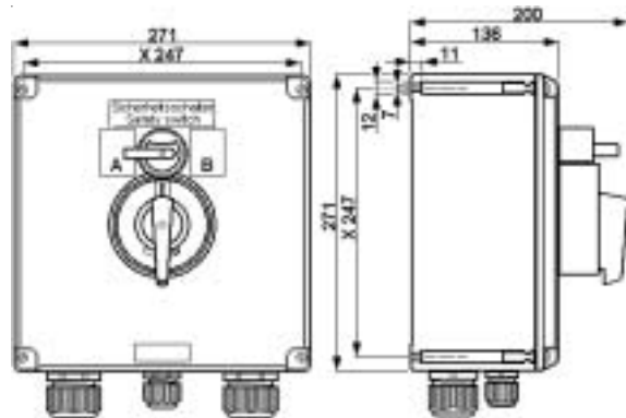
GHG 263 ..., 40A
