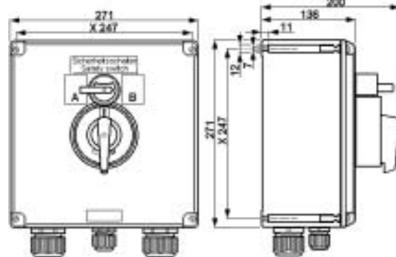
GHG 263 ..., 40A
