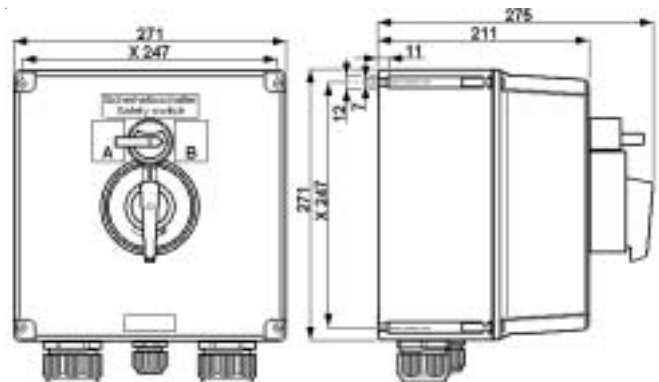
GHG 264 ..., 80A
