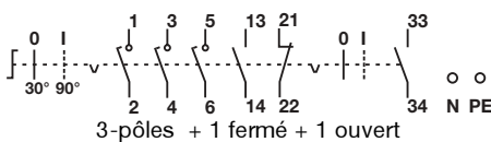
3-pôles + 1 fermé + 1 ouvert
