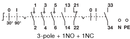
Wiring diagrams
