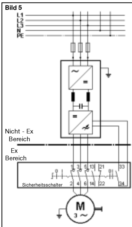
Anschlussbilder
