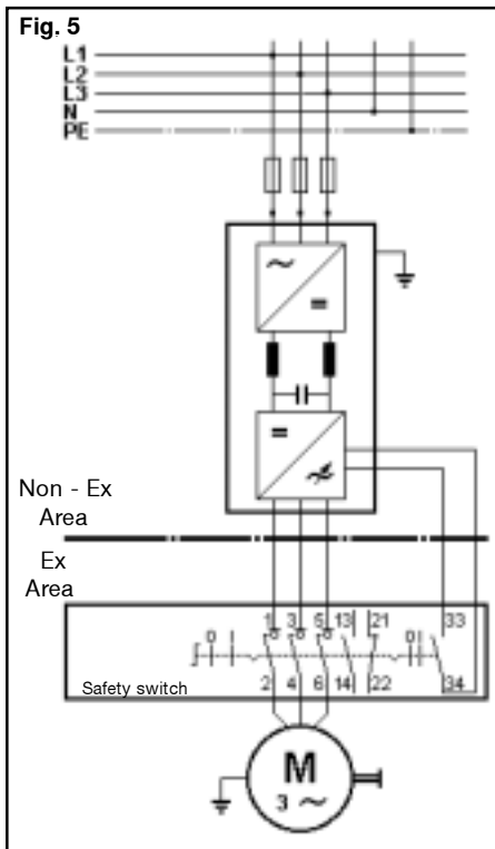
Wiring diagrams
