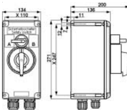
GHG 262 .., 20A
