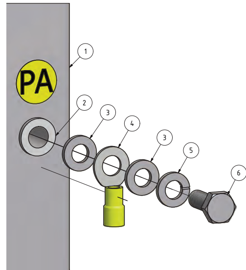
Potentialausgleich / equipotential bonding conductor / 等电位连接线 PA
