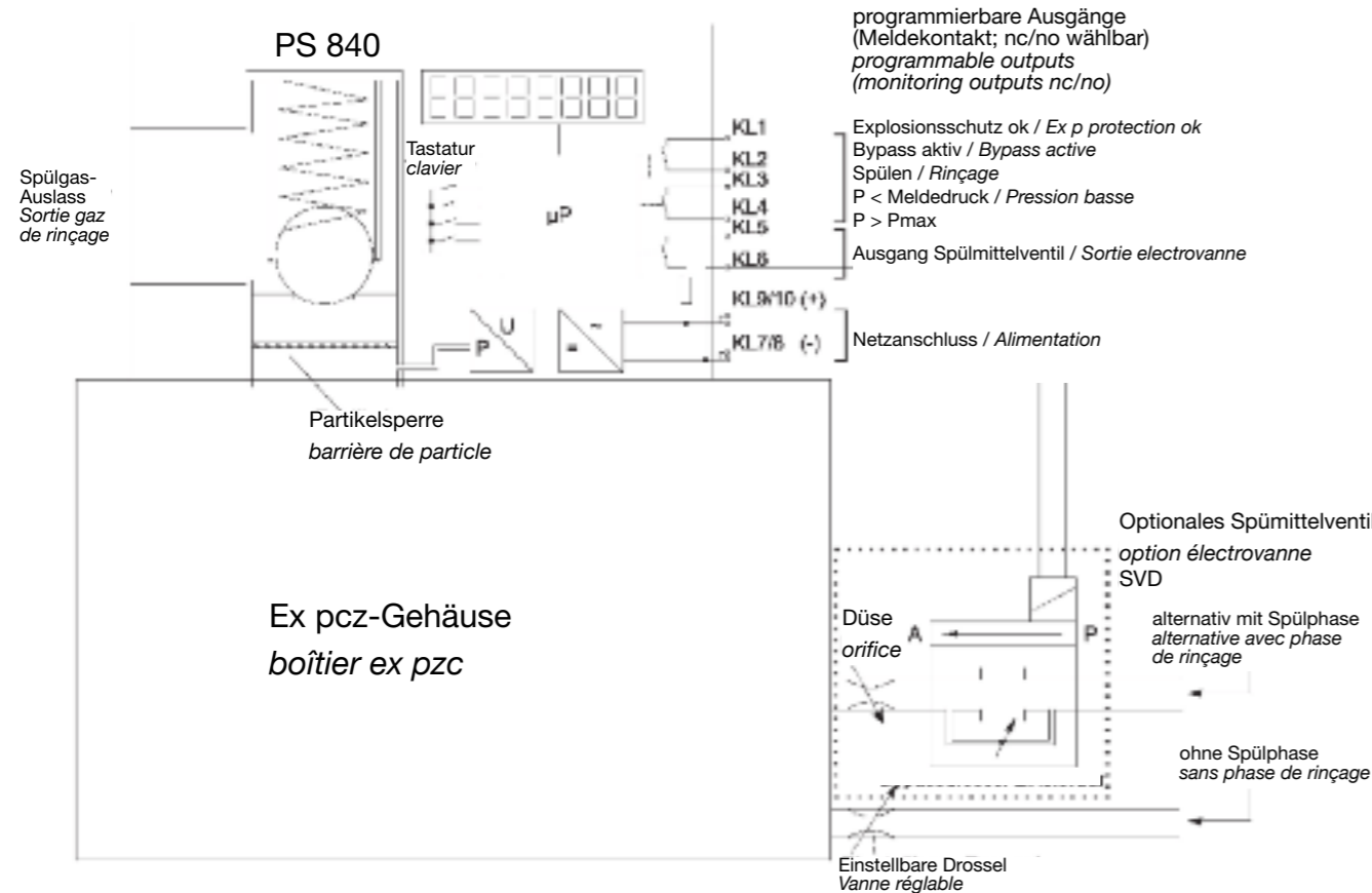
Abbildung 1 Blockschaltbild
