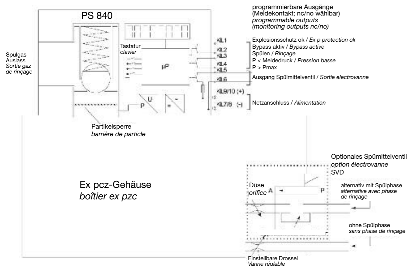
Abbildung 1 Blockschaltbild
