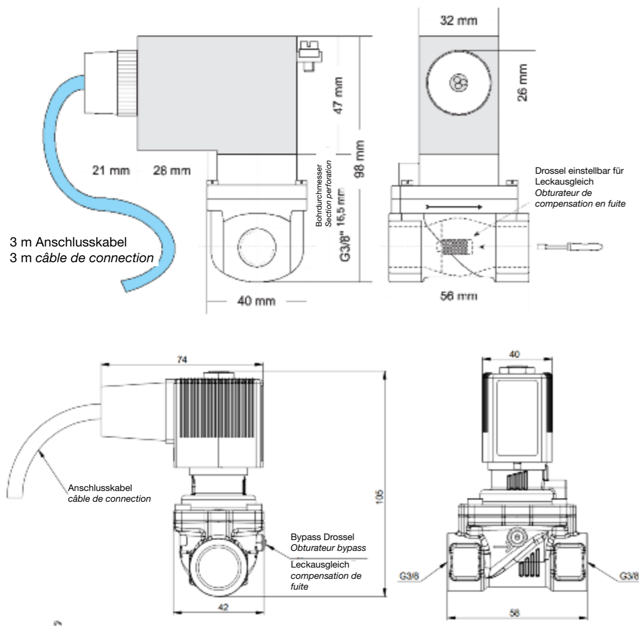
Abbildung 2: Spülmittelventil SVD.L.x-Axx (oben), SVD.L.x-Alxx (unten) Figur 2: Electrovanne SVD.Lx-Axx (en haut), SVD.L.x-Alxx (en bas)
