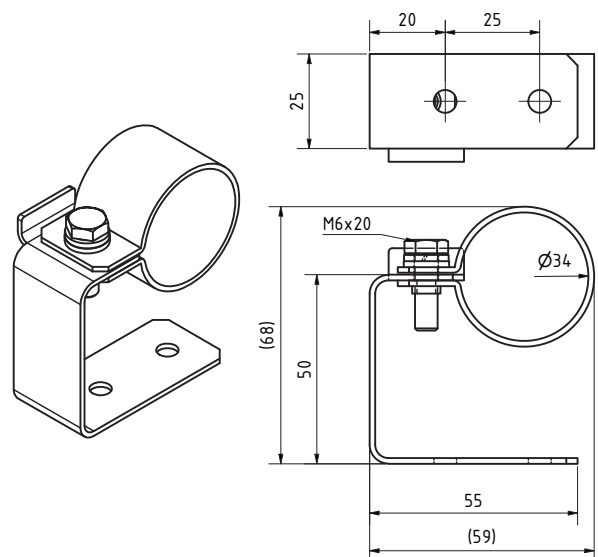
Abmessung / Dimension / Dimension
