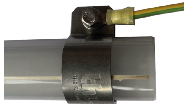
Mögliche Montagevariante mit Potentialausgleich Variante de montage possible avec liaison équipotentielle Possible installation variant with equipotential bonding
